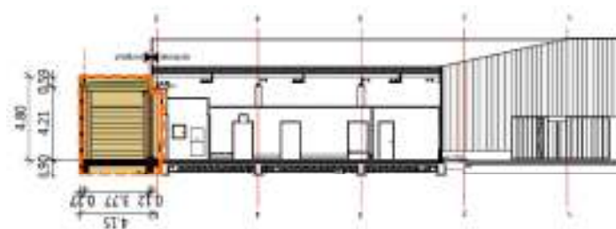
Prečni prerez načrtovanega prizidka (Studio Kalamar, avgust 2019)
