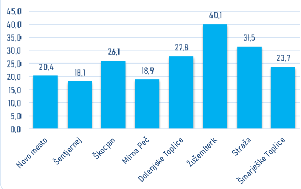
Graf 6: Vodne izgube v % po občinah
