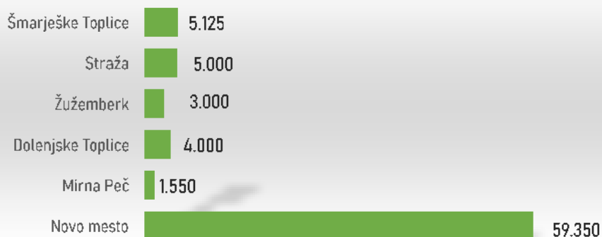
Graf 17: Skupno število populacijskih enot (PE) po občinah
