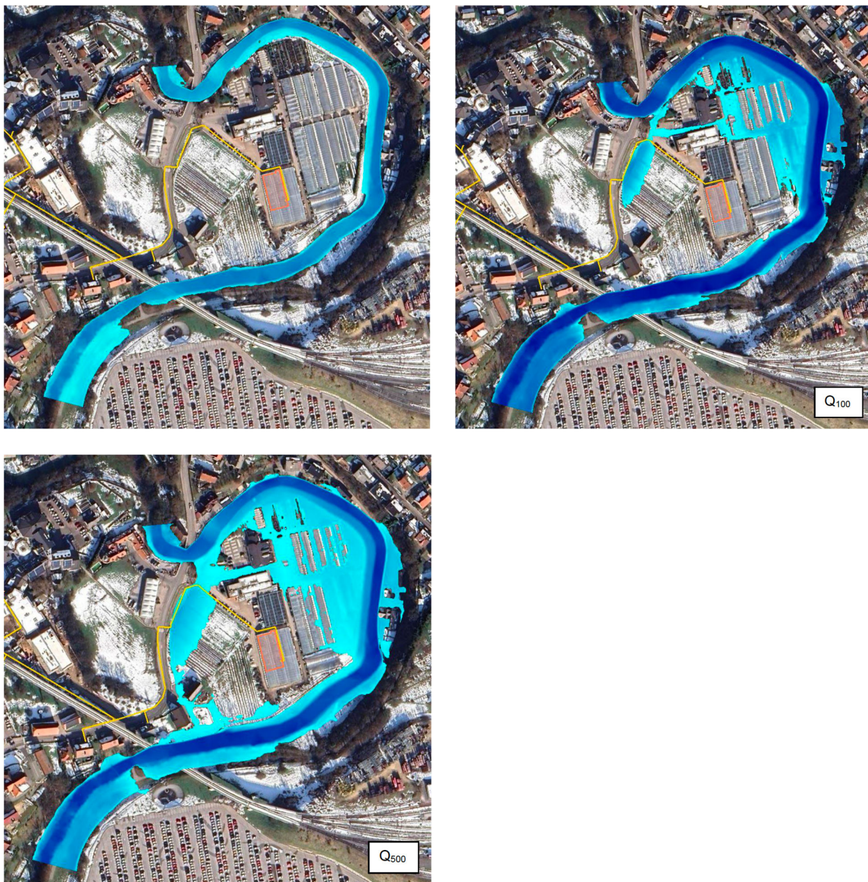
Slika 8: Prikaz obsega poplav obstoječega stanja ob nastopu visoke vode Q_{10} , Q_{100} in Q_{500}
