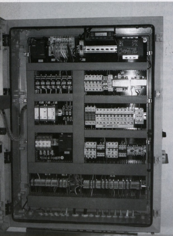
Krmilna omara v črpališču
